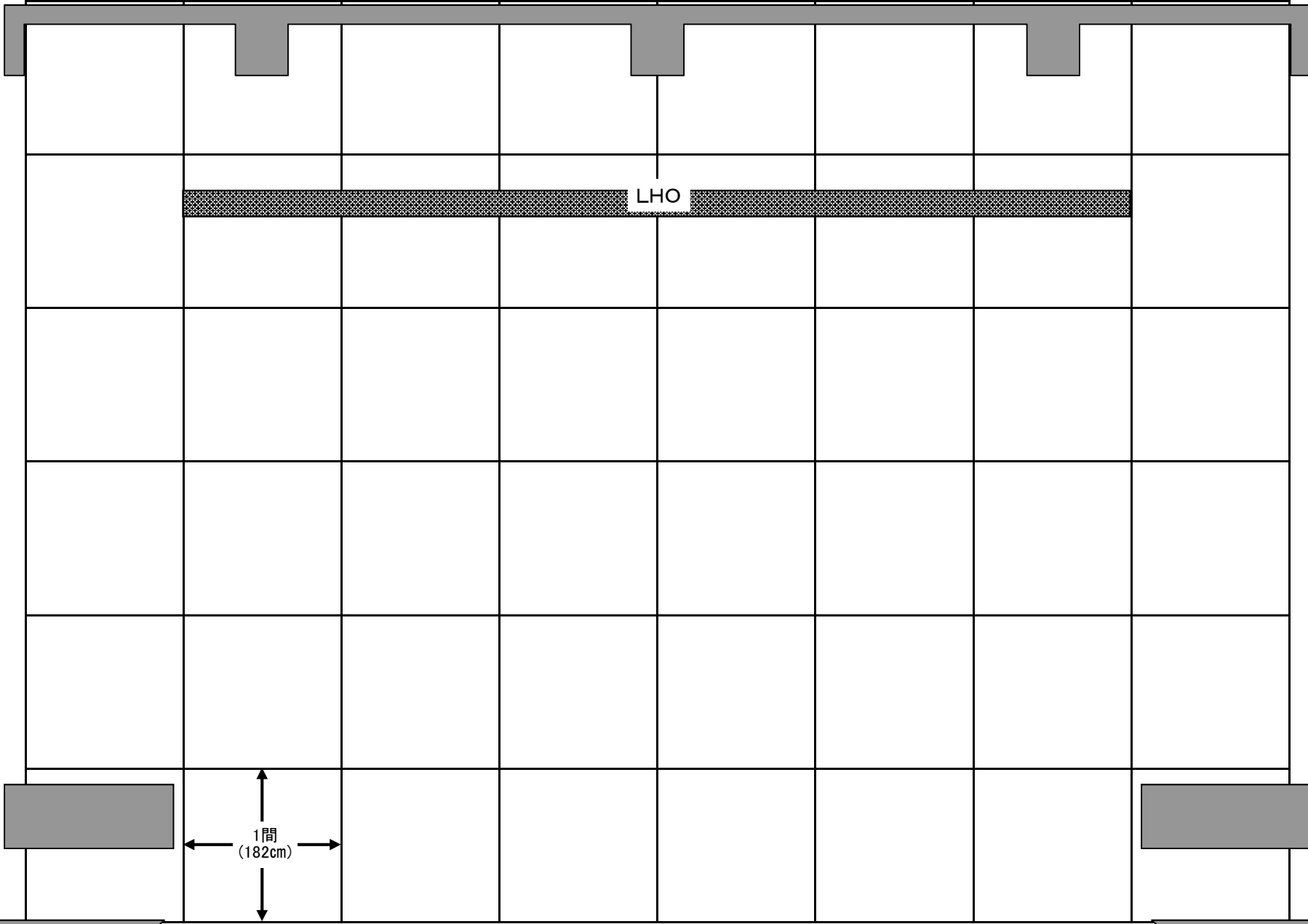
江南市民文化会館 小ホール 平面図
